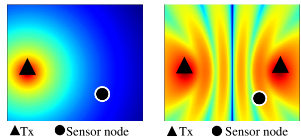
図1: 単一の送電アンテナを用いた電波電力伝送 図2: 複数の送電アンテナを用いた電波電力伝送
