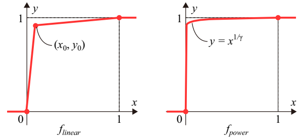
図 3 指示関数の近似に用いる微分可能な関数の候補.
