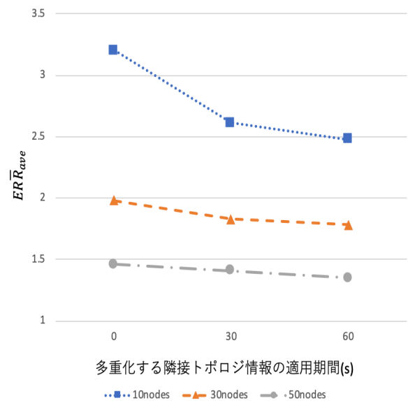
図 7 SmartFinder の従来手法と提案手法の平均誤差比較
