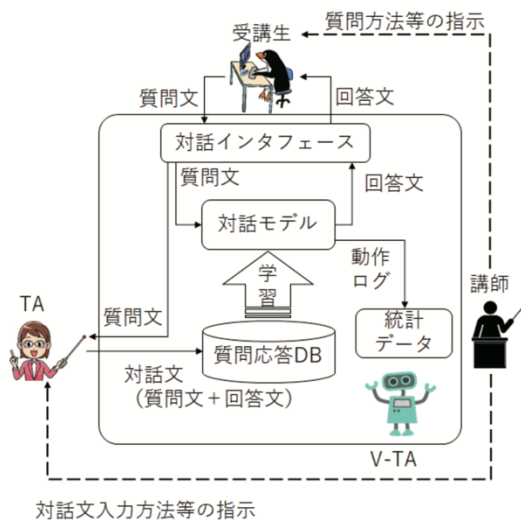
図 1: 対話システム「V-TA」の全体像 [3]
