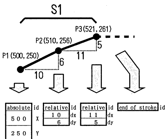
図5 図4 (b) に示した点レコード P1, P2, P3 の詳細な構造と内容例
