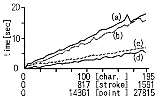
図10 ストロークファイルの入出力時間。char., stroke, point はそれぞれ字, 画, 点の数を意味する。(画と点の数は (a) (b) の場合を示す) (a) 実画と虚画の出力時間 (b) 実画と虚画の入力時間 (c) 実画だけの出力時間 (d) 実画だけの入力時間
