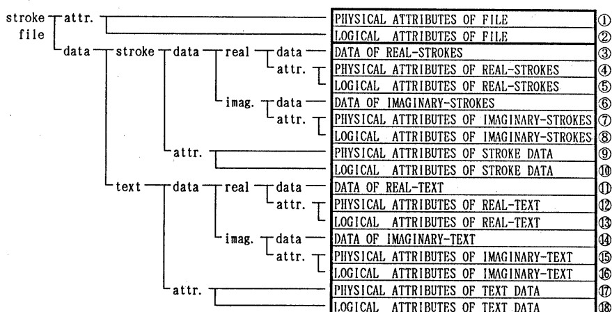
図3 ストロークファイル全体の構成（右側の枠内）と構成要素の階層構造（左側の木）．'attr.'は'attributes'の，'imag.'は'imaginary'のそれぞれ省略形を示す．枠内の大文字の部分はその部分がより細かな要素から構成されていることを示す．
