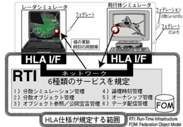
図 1 HLA の概要 [9]
