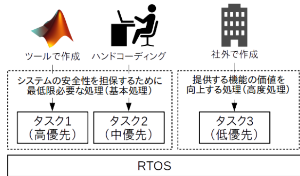
図 1 統合前アプリの概要
