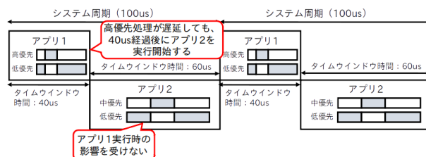
図 3 TDMA スケジューリング
