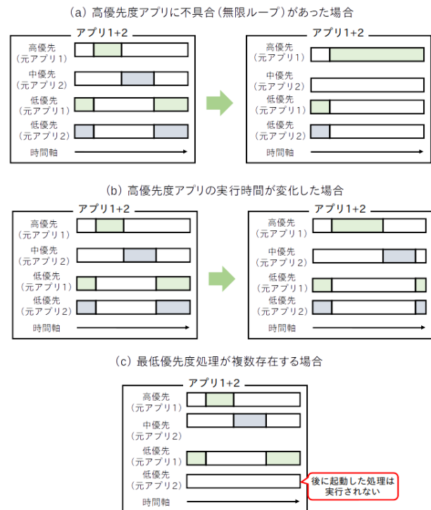
図 2 優先度ベースのスケジューリングによる統合の問題
