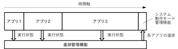
図 5 ランタイムの構成
