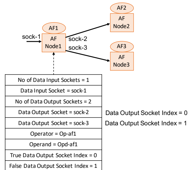
AFC Daemonがもつ管理テーブルの一部
