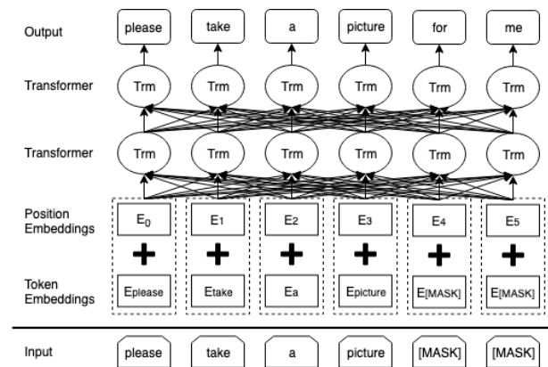
図 3 BERT
