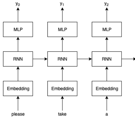
図 2 RNNLM
