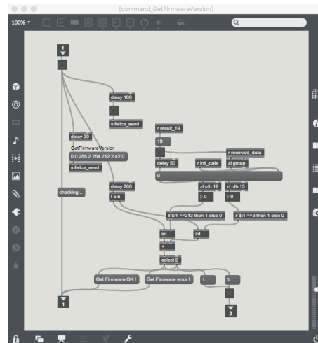
図13 「command_GetFirmwareVersion」サブパッチ.
