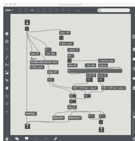
図12 「command_Reset」サブパッチ.
