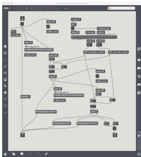
図14 「command_RFConfiguration」サブパッチ.
