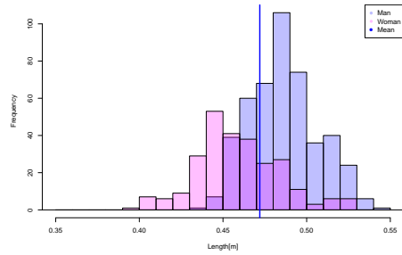
図4 ArmLength の分布
