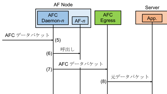
図 11 AFC 設置のシーケンス後半部分
