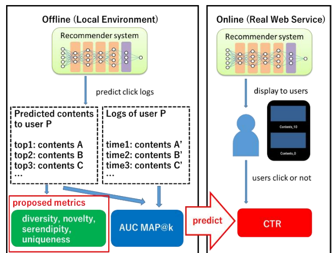
図1 本研究の概念図。提案するオフライン検証指標により、CTR に近い評価を行うことを目指す。
