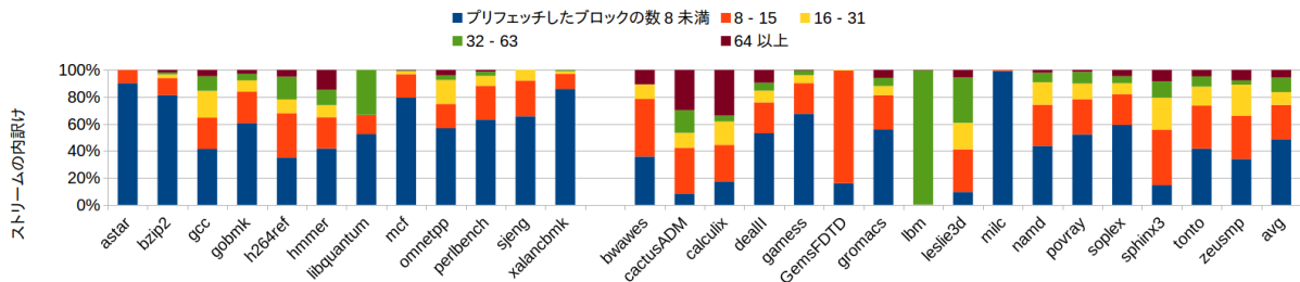
図 12 学習できなかったストリーム数の分布 (ストリームテーブル 32 エントリ)
