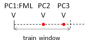
図 14 FML とプリフェッチ方向を決める二つのミス
