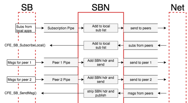
図 3 SB と SBN によるプロセッサ間メッセージ通信例
