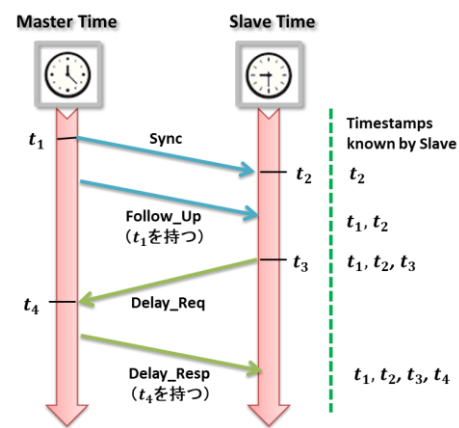
図 2 時刻同期の情報伝送と伝播遅延の計測
