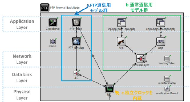
図 5 車載 ECU ノードのシミュレーションモデル
