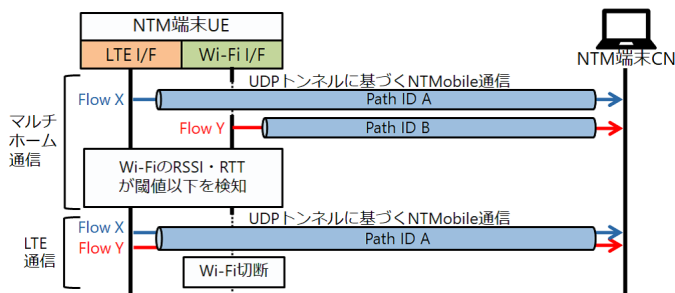
図 7 シングルホームの CN に対して UE がマルチホームから LTE にハンドオーバーする場合の通信シーケンス (パターン 2)
