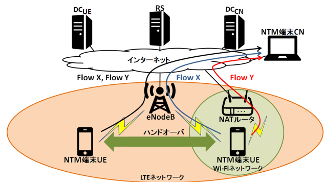
図 5 NTMobile における IP Flow Mobility の概要
