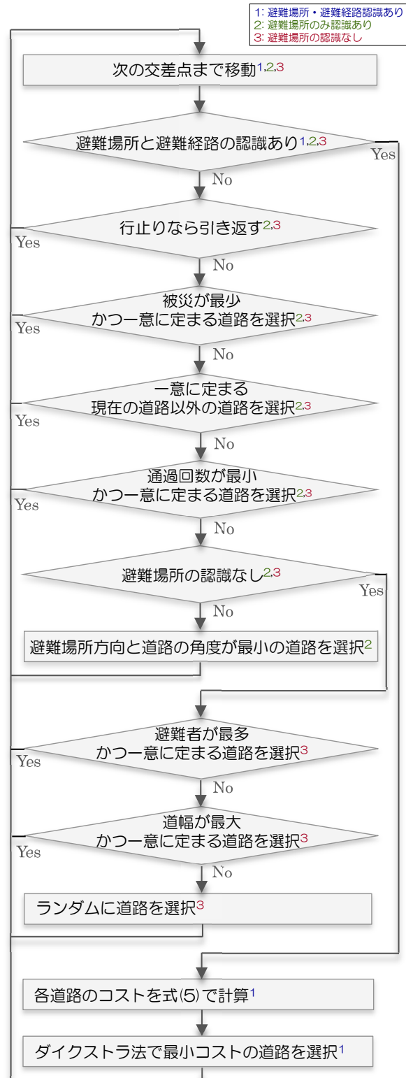
図1 経路選択モデルのアルゴリズム Figure 1 The algorithm of route choice model.
