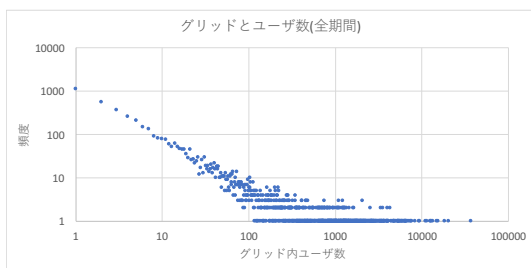
図3 グリッドごとのユーザー数
