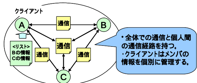
図1. グループ内部構成モデル図
