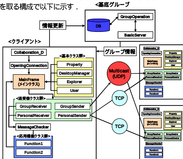
図 9. システム全体のクラス構成図
