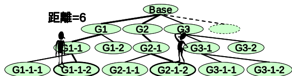
図 7. グループ間距離モデル図
