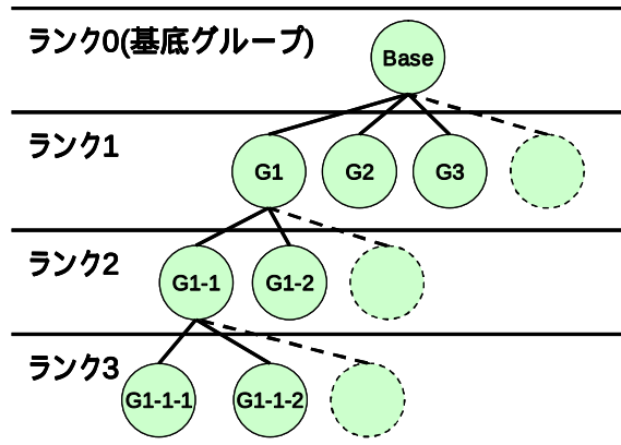
図6. グループのランク
