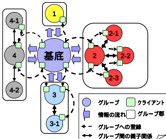
図5. 基底グループを中心とした相互関係図
