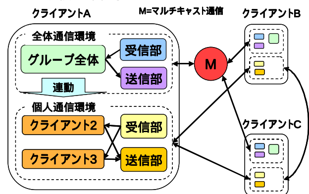
図2. グループの内部構成モデル図
