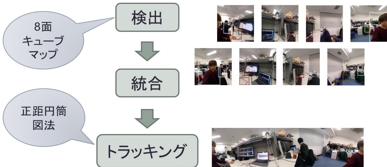
図 1 提案手法の流れ
