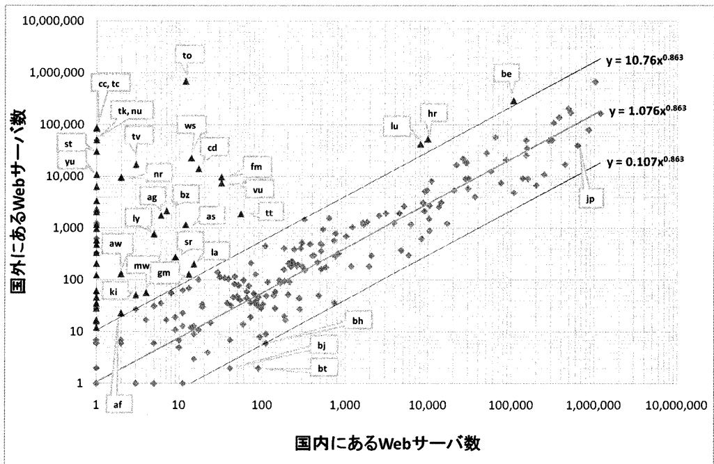
図 4 自国内 Web サーバ数と国外 Web サーバ数の適正範囲とアンバランスな ccTLD
