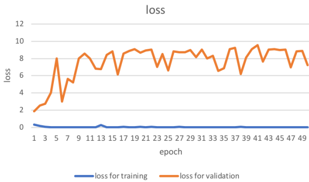
図 7 検証 1 の損失
