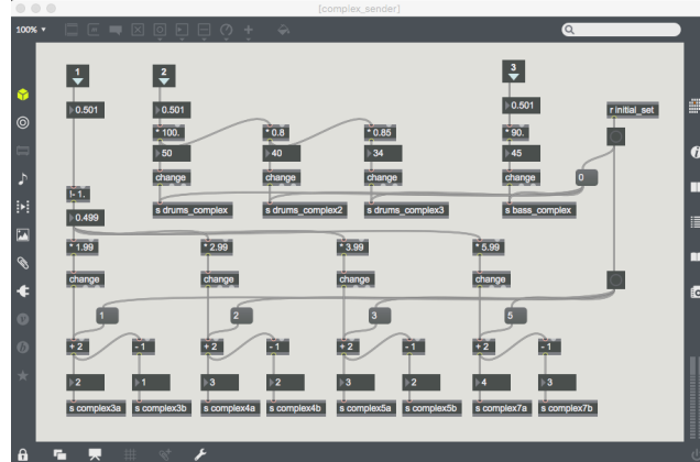
図 35 「メロディーノート重み付け」生成パッチ Figure 35 Melody Notes Random-Weight.
