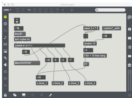
図 13 「chord_get」サブパッチ Figure 13 chord_get.
