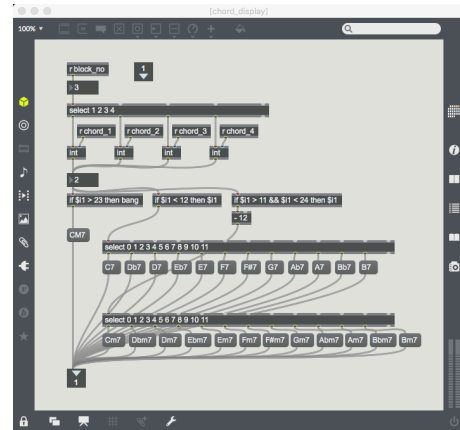
図 14 「chord_display」サブパッチ Figure 14 chord_display.
