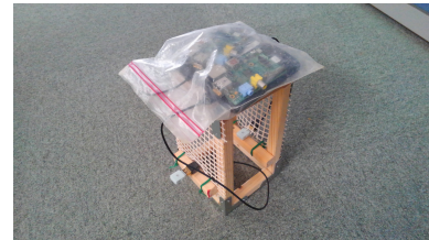
図 4 無線通信特性測定用機材
