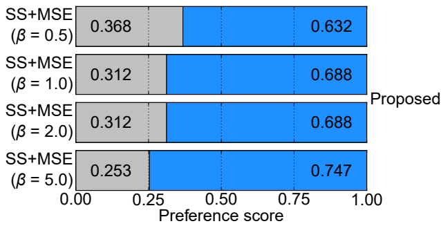
図 4 合成音声品質に関するプリファレンススコア (SNR = 0 dB) Fig. 4 Preference scores on synthetic speech quality (SNR = 0 dB).
