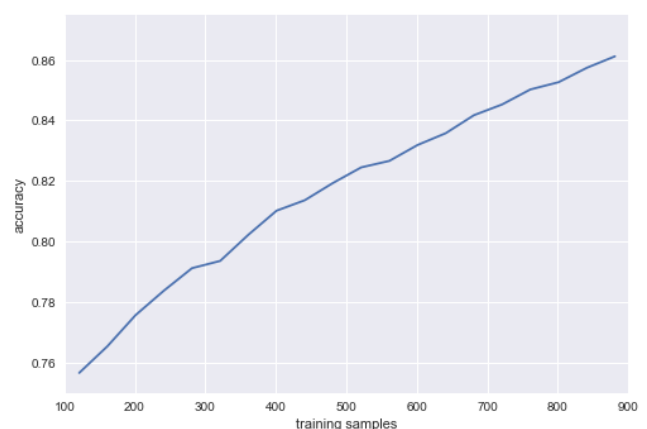
図 3 学習データサイズ (training samples) と精度 (accuracy) の関係
