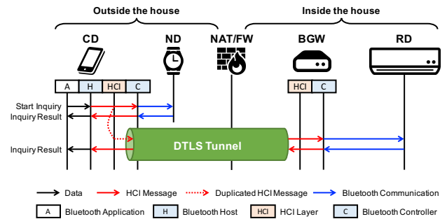
図 6 Bluetooth 通信シーケンス
