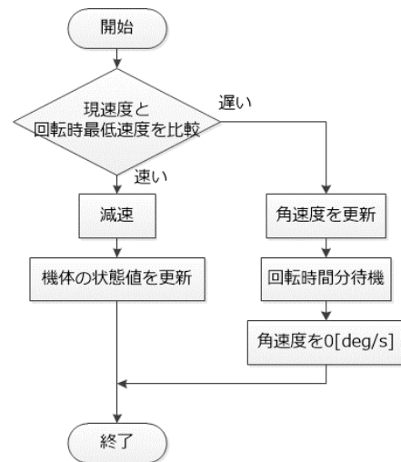
図 12 回転制御のフローチャート
