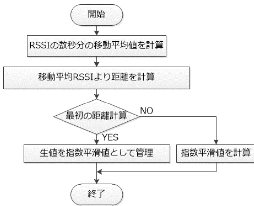
図 8 距離推定のフローチャート
