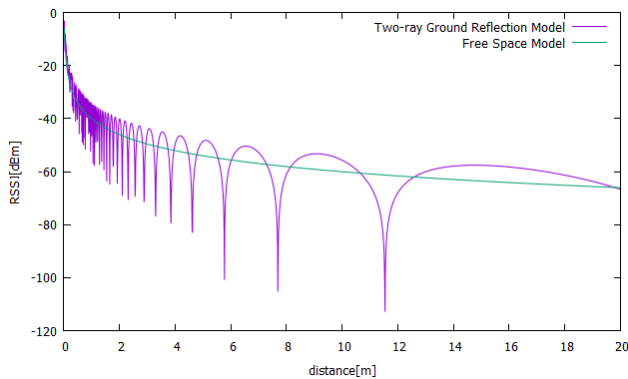
図 5 電波の減衰特性
