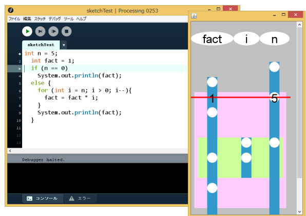
図 2. PDE と試作ツールの実行画面例
