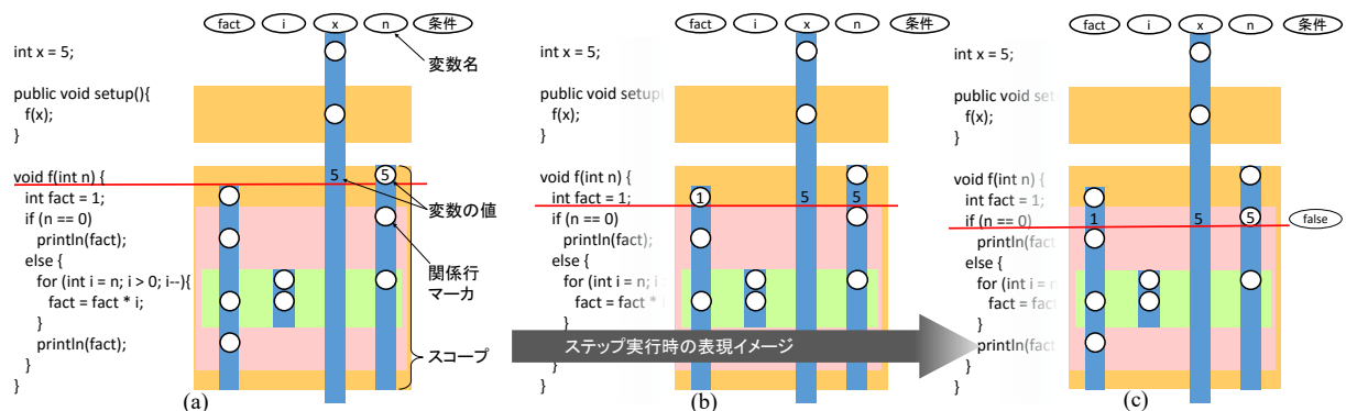
図 1. 独自の図表現によるプログラム構造の可視化
