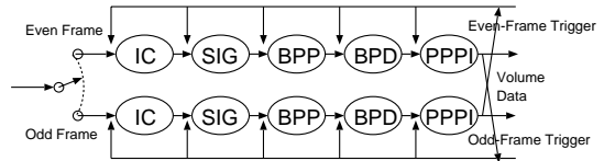
図 13 複数スレッドによるパイプライン処理の実装
