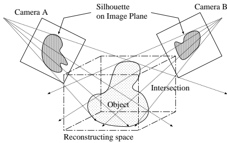
図 1 視体積交差法の概念図
