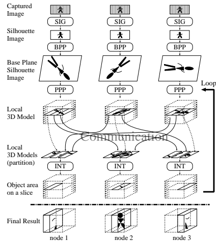
図 9 ローカルシルエット分割法の処理の流れ
