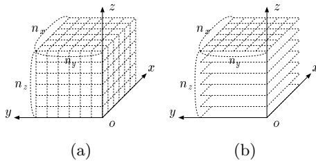
図 6 3次元空間の分解法：(a) 3次元ボクセル空間，(b) 平行平面群への分割
