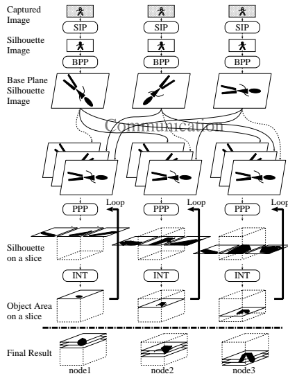
図 10 基準シルエット多重化法の処理の流れ
