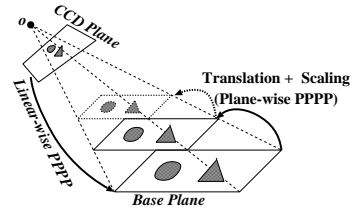
図 8 面単位の平面間透視投影
