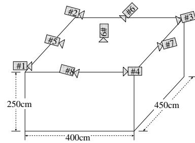
図 11 カメラの配置
