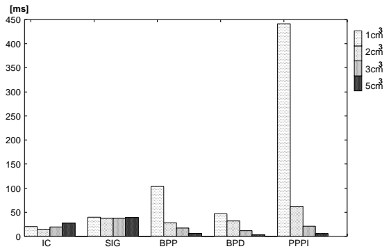
図 17 各ステージでの処理時間（50 フレームの平均処理時間） Fig. 17 Average elapsed time in processing stages for 50 frames.
