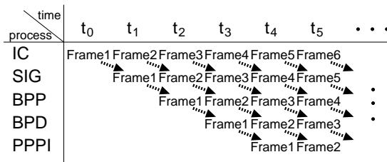
図 12 各ノード PC でのパイプライン処理
