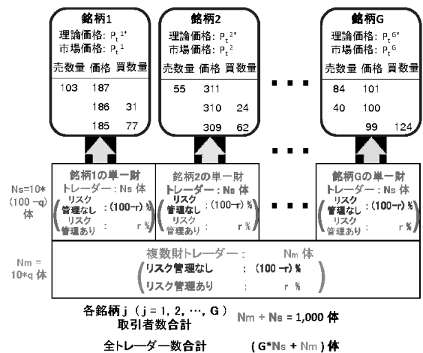
図 1 複数財資産市場の構造
