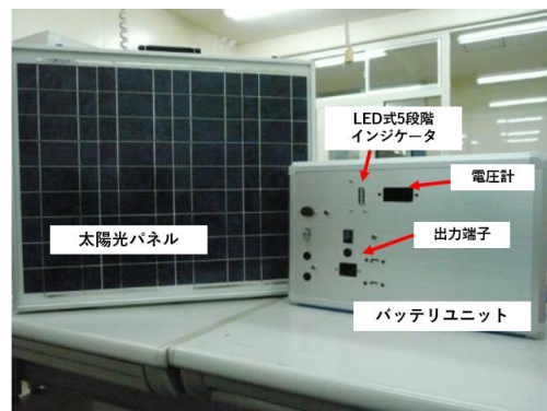
図 2 実際に開発した太陽光発電システム
