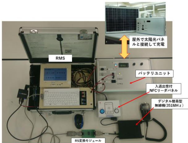
図7 RMS(避難所管理システム)のプロトタイプシステム
