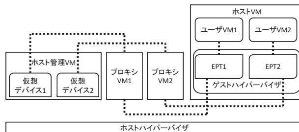
図 5 プロキシ VM を用いたユーザ VM への仮想デバイスの提供
