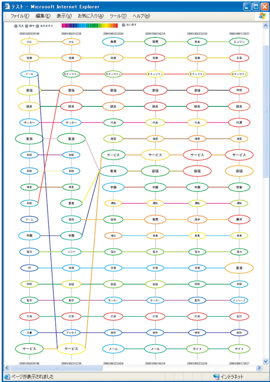
図 7 T-Scroll のスクリーンショット (1 日刻み) Fig.7 Screenshot of T-Scroll (daily basis).
