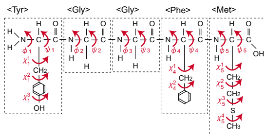
図 11 Met-enkephalin の構造
