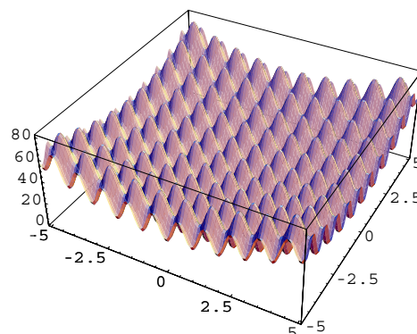
図 1: Rastrigin 関数の概形
