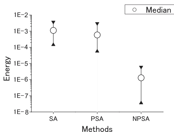
図 3: SA, PSA, NPSA の探索性能の比較
