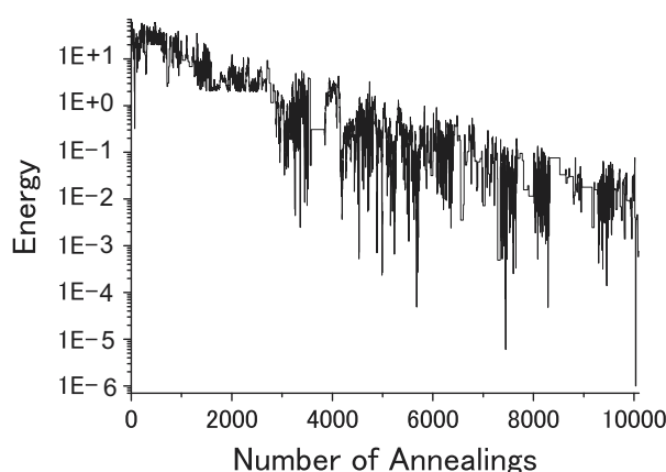
図 4: NPSA のエネルギー履歴
