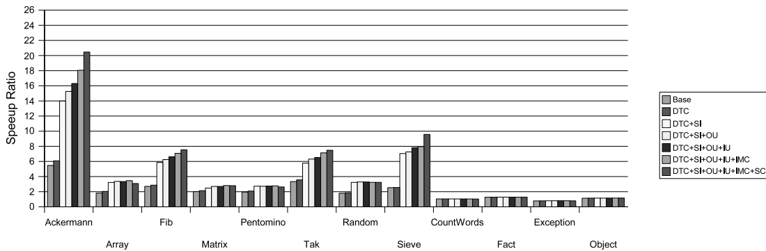
図 12 x86 プロセッサ上でのマイクロベンチマークの評価結果 Fig. 12 A result of micro benchmark tests on an x86 processor.
