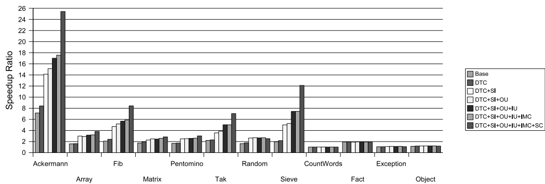
図 13 x86_64 プロセッサ上でのマイクロベンチマークの評価結果 Fig. 13 A result of micro benchmarks tests on an x86_64 processor.
