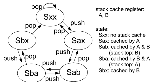
図 5 スタックキャッシングの状態遷移図 Fig. 5 A state transition diagram of stack caching.
