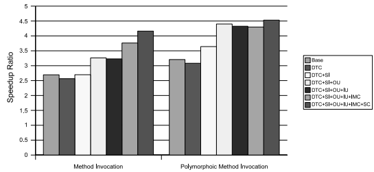
図 11 メソッド起動速度の評価
