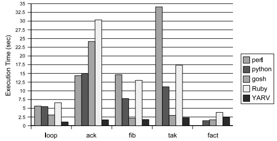
図 15 他言語との速度比較
