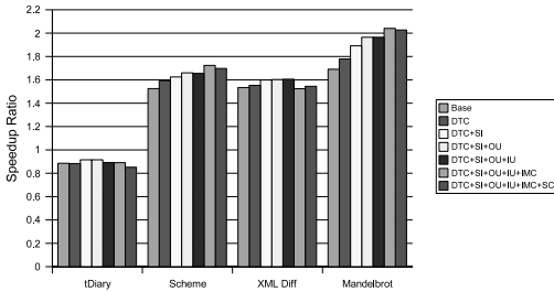
図 14 マクロベンチマークの評価結果
