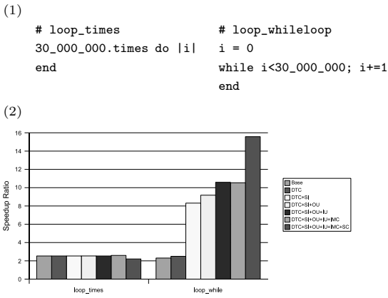
図 10 繰り返し実行速度の評価
