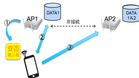
図 2: アプリケーション概要
