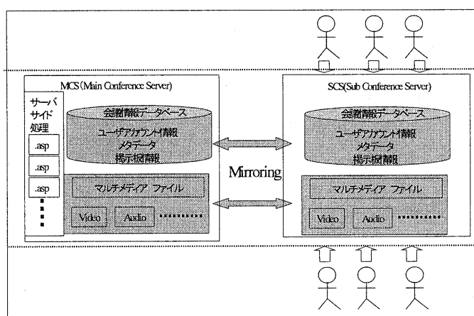
図4 ASSIST のフレームワーク
