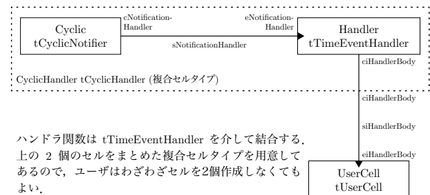
図 6 タイムイベント通知コンポーネントにハンドラ関数を結合する方法
