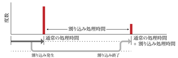
図 7 ヒストグラムを用いて割り込み処理時間を計測する方法
