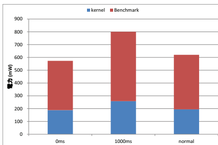
図 7 消費電力
