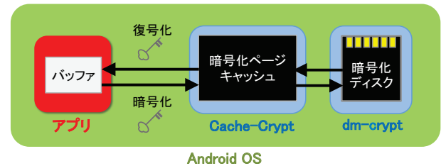
図 1 ファイルの読み書きの流れ
