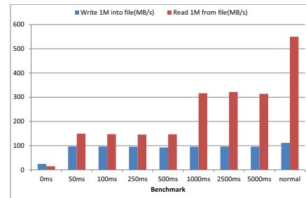
図 3 ファイル読み書きの性能
