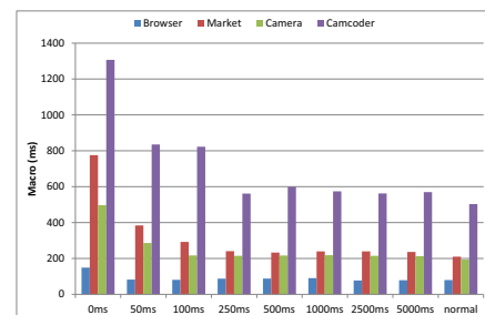
図 5 実アプリの性能
