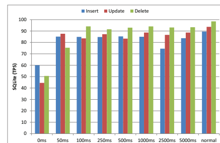
図 4 SQLite の性能
