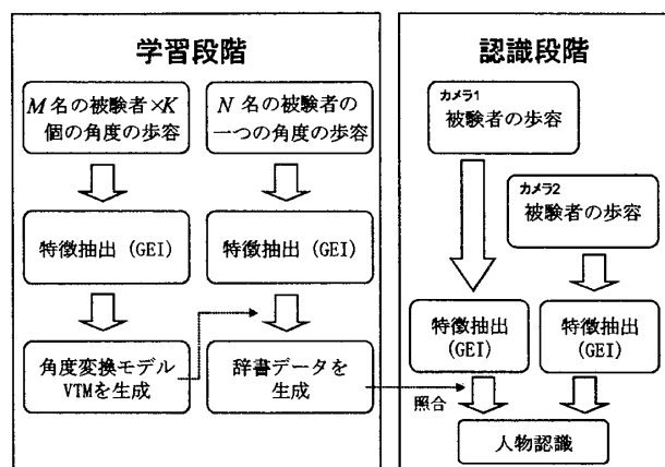
図 1: 提案手法の流れ (2台カメラを用いる場合)
