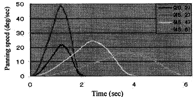
図8 ロボットカメラによるカメラワークの再現 (カッコ内は、パンニング角度とショット時間)
