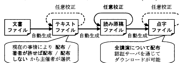
図1. 点訳機能つき講演原稿受付システムの流れ
