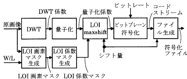
図2 LOI 符号化方式
