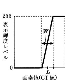
図1 画素値・表示輝度値変換
