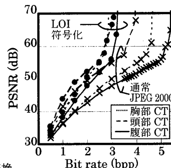
図3 LOI 符号化による PSNR 特性改善効果
