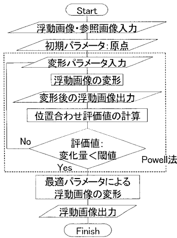
Fig.3 位置合わせ処理の流れ
