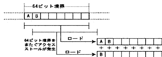
図 2 プロセッサ・ストールが発生する演算の例：要素 A・B 間でパックド・データ演算を行う場合、パックド・データ内での A,B の位置を合わせるために 64 ビット境界をまたぐアクセスが発生し、プロセッサがストールする。
