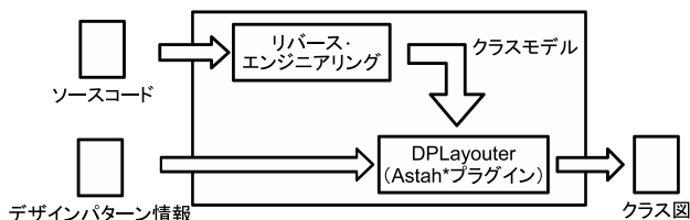
図1: DPLayerのシステム構成図
